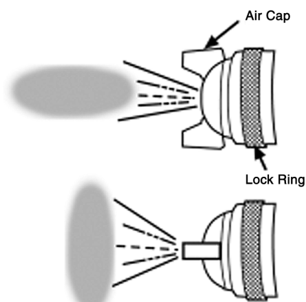
(Dwg. TP2053)
