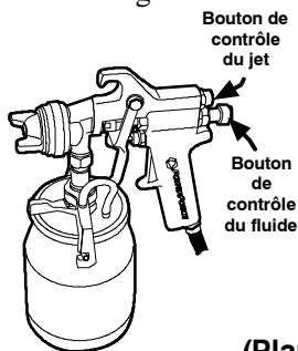
(Plan TP2044)
