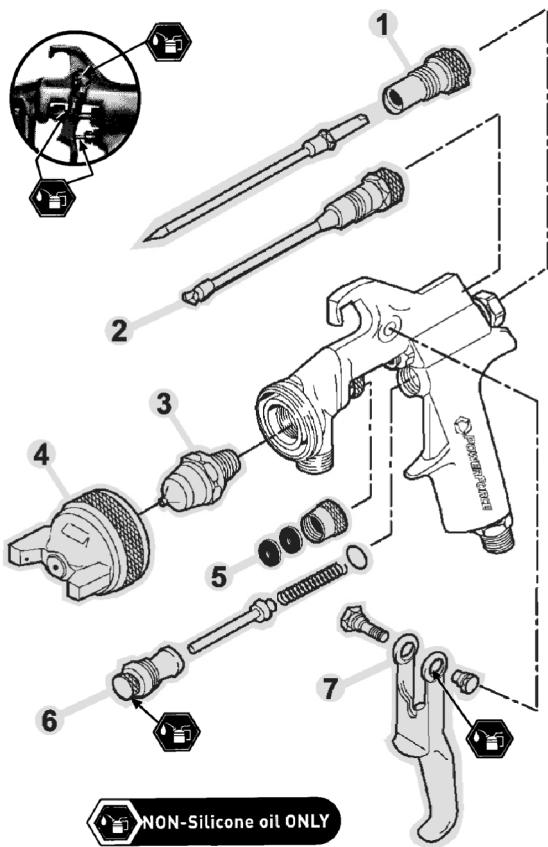
(Dwg. TP1954)
